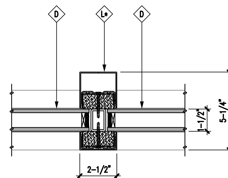
10 DOOR TOP RAIL DTL 3\" = 1'-0"
