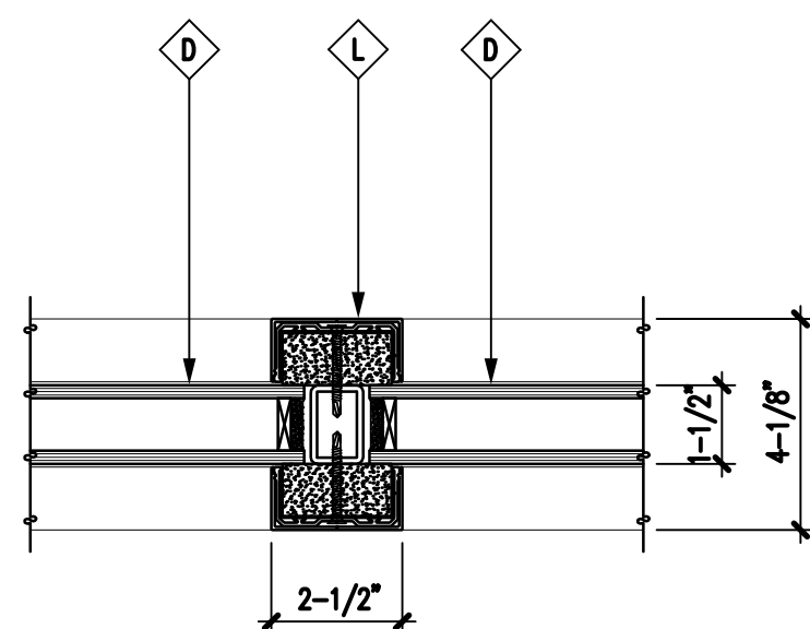
6 JAMB DTL 3\" = 1'-0"
