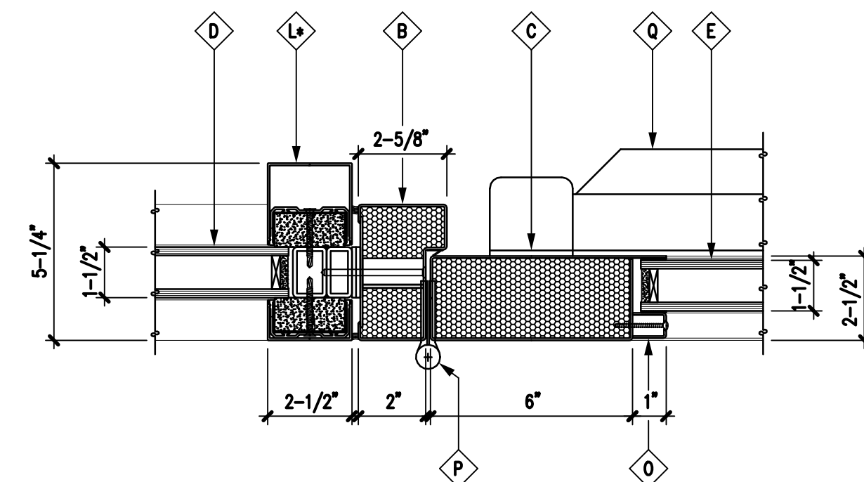
8 DOOR JAMB @ HINGE DTL 3\" = 1'-0"
