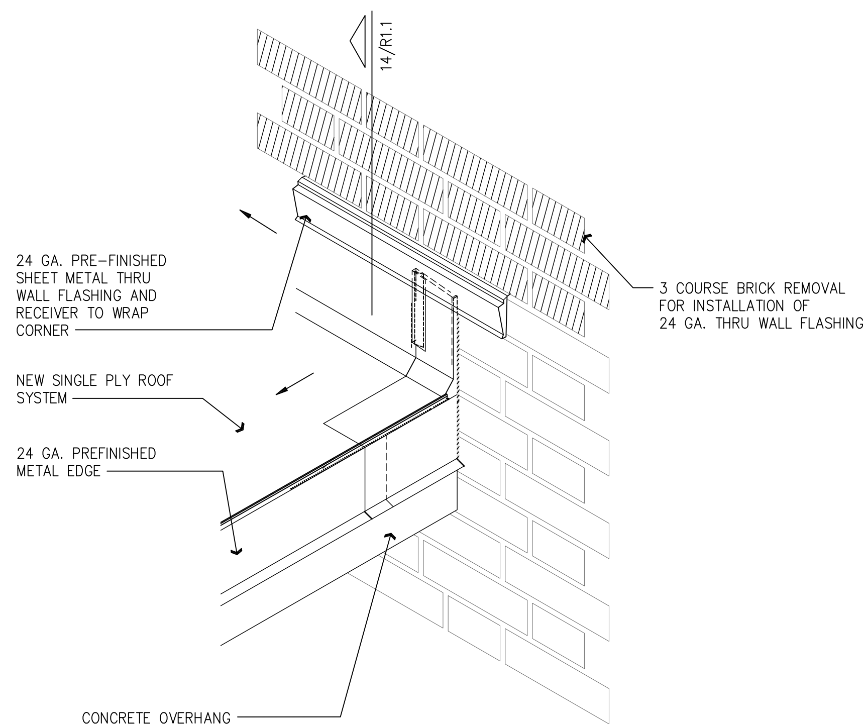
10 EDGE CONDITION DETAIL
