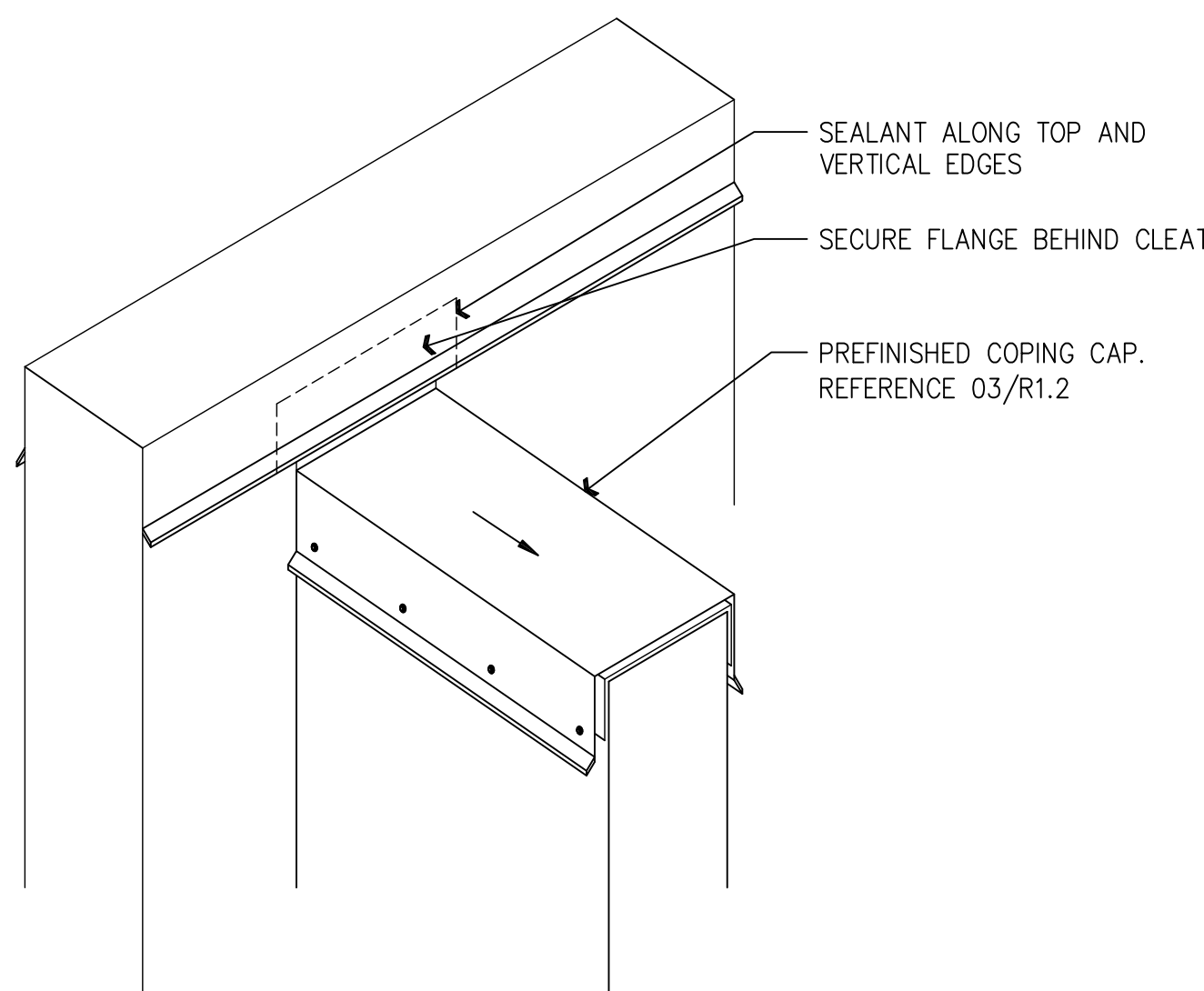
08 EDGE METAL FLASHING DETAIL
