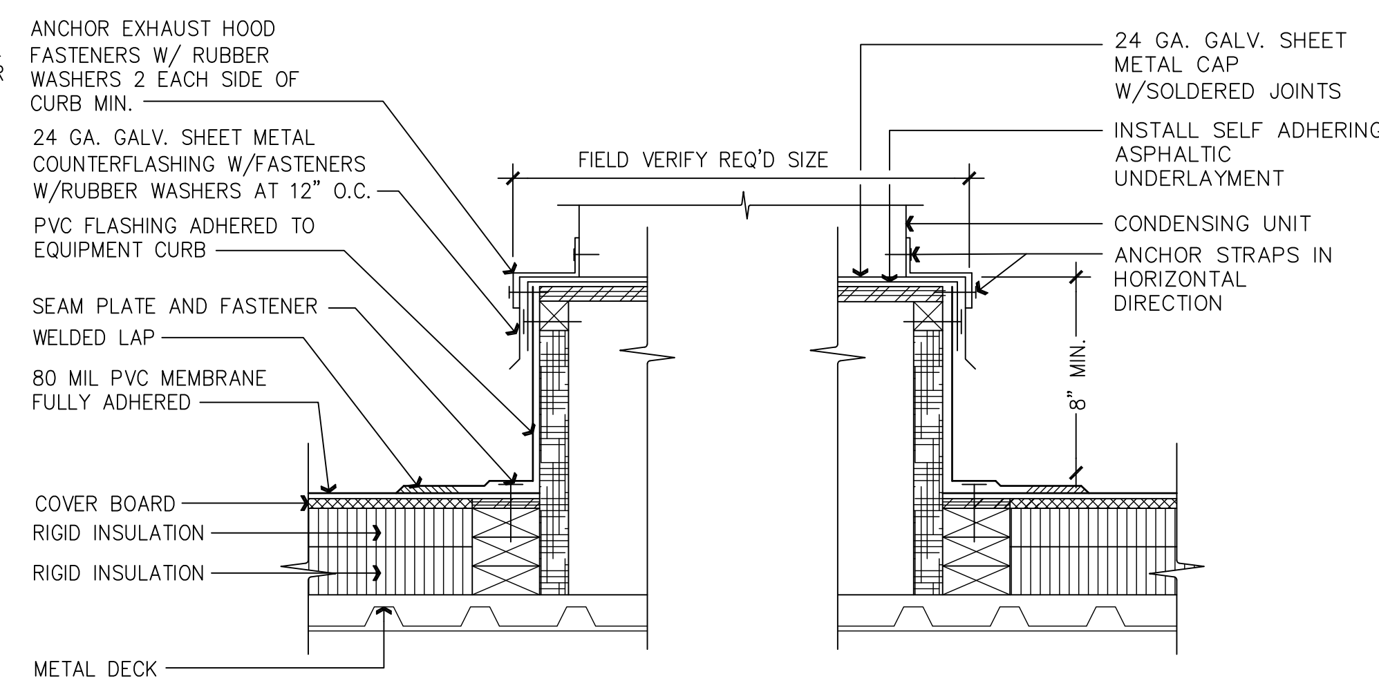
09 CONDENSING UNIT DETAIL SCALE: 1-1/2" = 1'-0"
