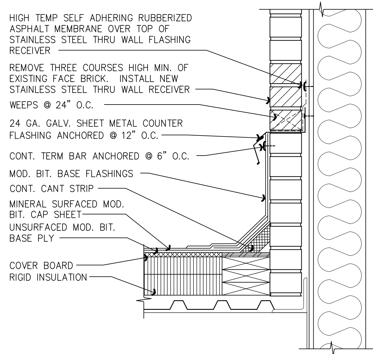
14 RISE WALL DETAIL SCALE: 1-1/2" = 1'-0"
